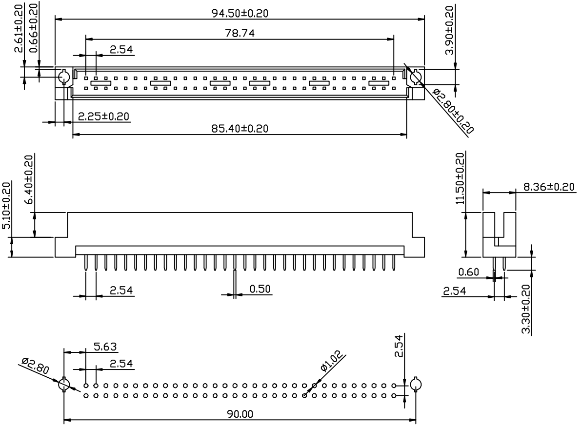
P.C.B LAYOUT
